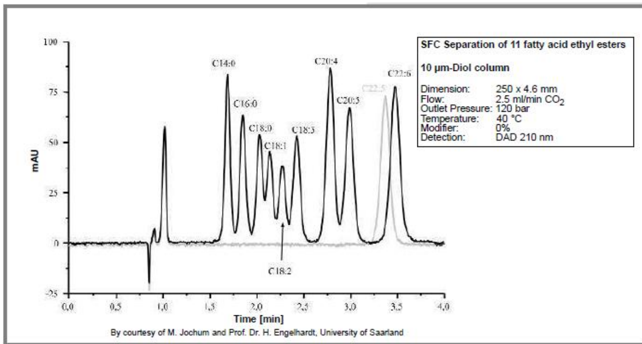
超临界流体色谱分离 11 种脂肪酸乙酯
